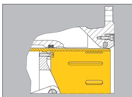
Tipo SZ con camisa ranurada Type SZ with slotted cylinder
