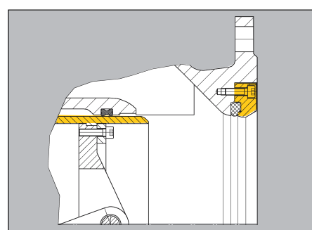
Asiento tipo E Seat type E
