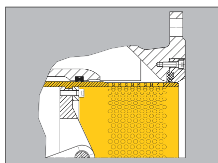
Tipo LH con camisa perforada Typ LH with anti cavitational multiple orifice cylinder
